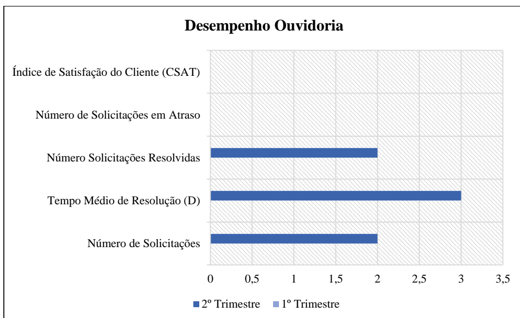
Gráfico 5: Desempenho Ouvidoria
