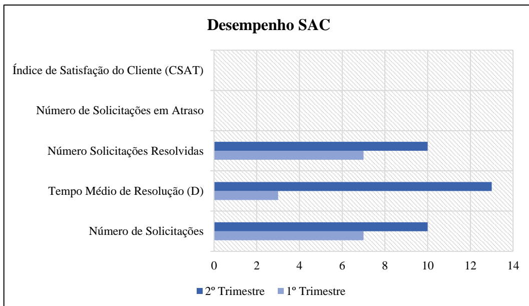
Gráfico 4: Desempenho SAC
